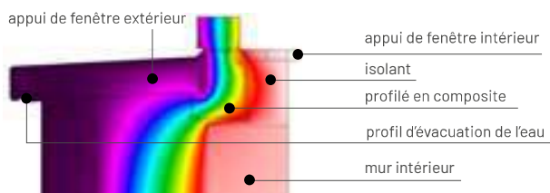
Appui de fenêtre
