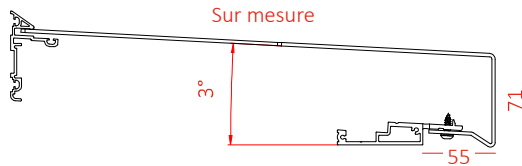
Appui de fenêtre en aluminium
