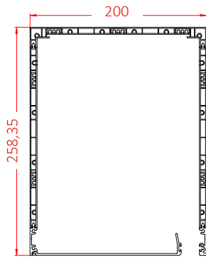
Caisson, vue de côté
